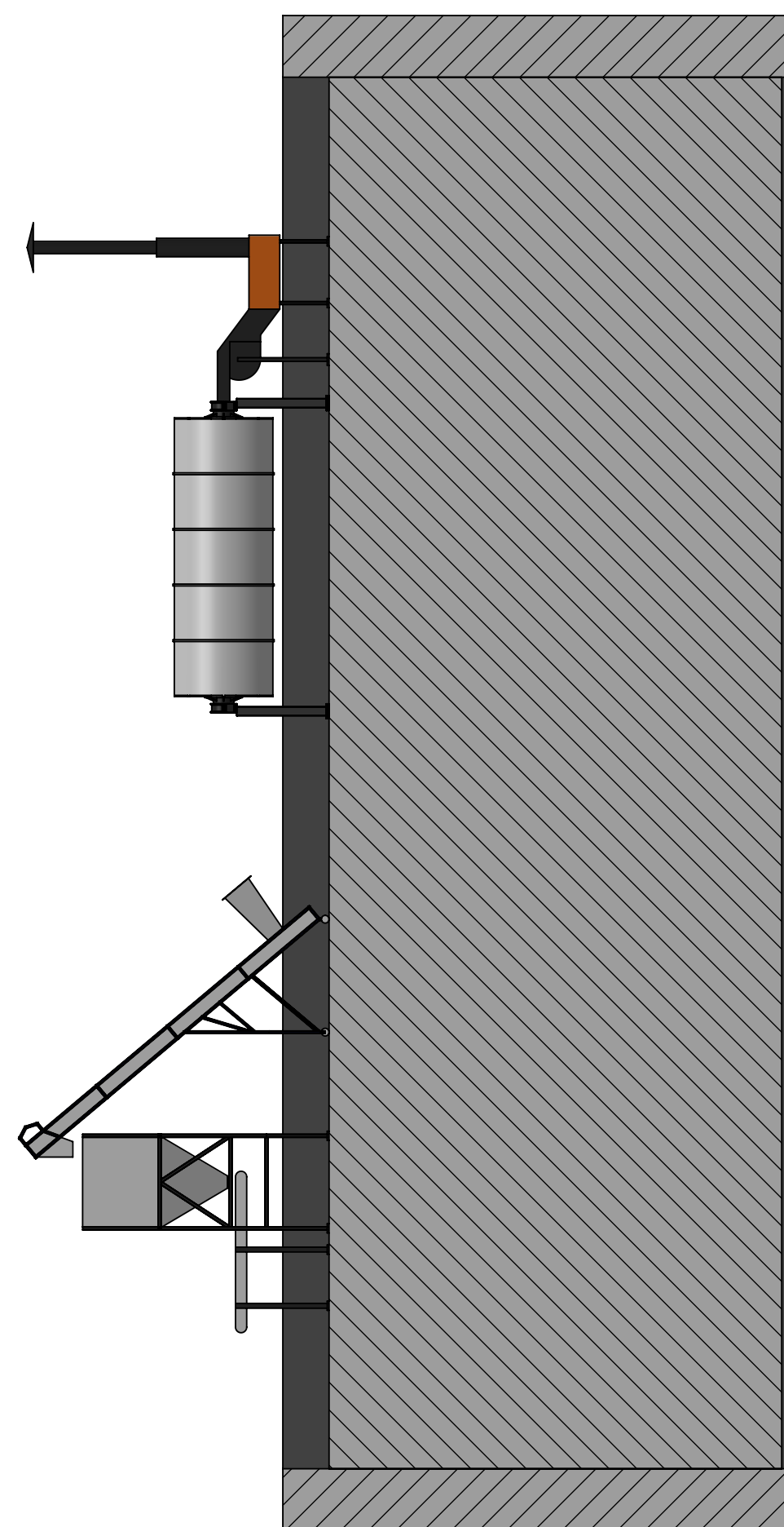
SEÇÃO B-B
